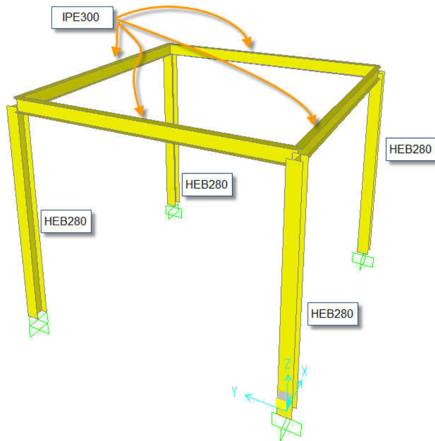
Figura 24. Perfiles de acero seleccionados para el análisis.
