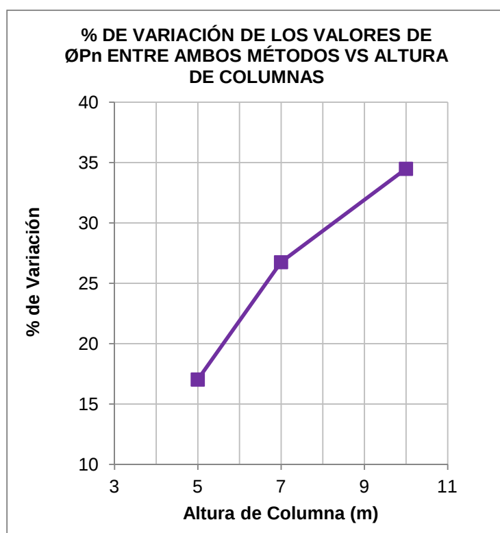
Gráfica 6. Porcentaje de Variación de \phi P_n entre ambos métodos vs altura de columna
