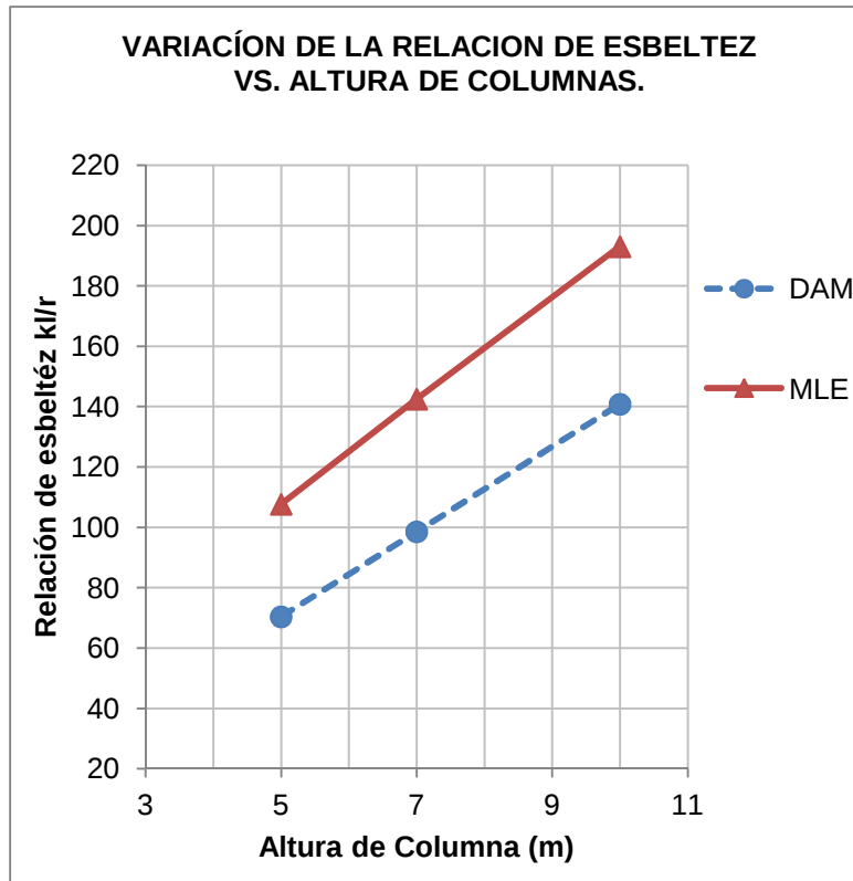
Gráfica 4. Relación de esbeltez vs altura de columnas.
