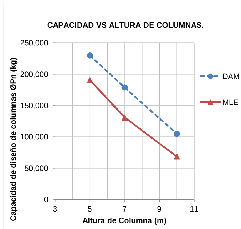
Gráfica 5. Capacidad vs altura de columna
